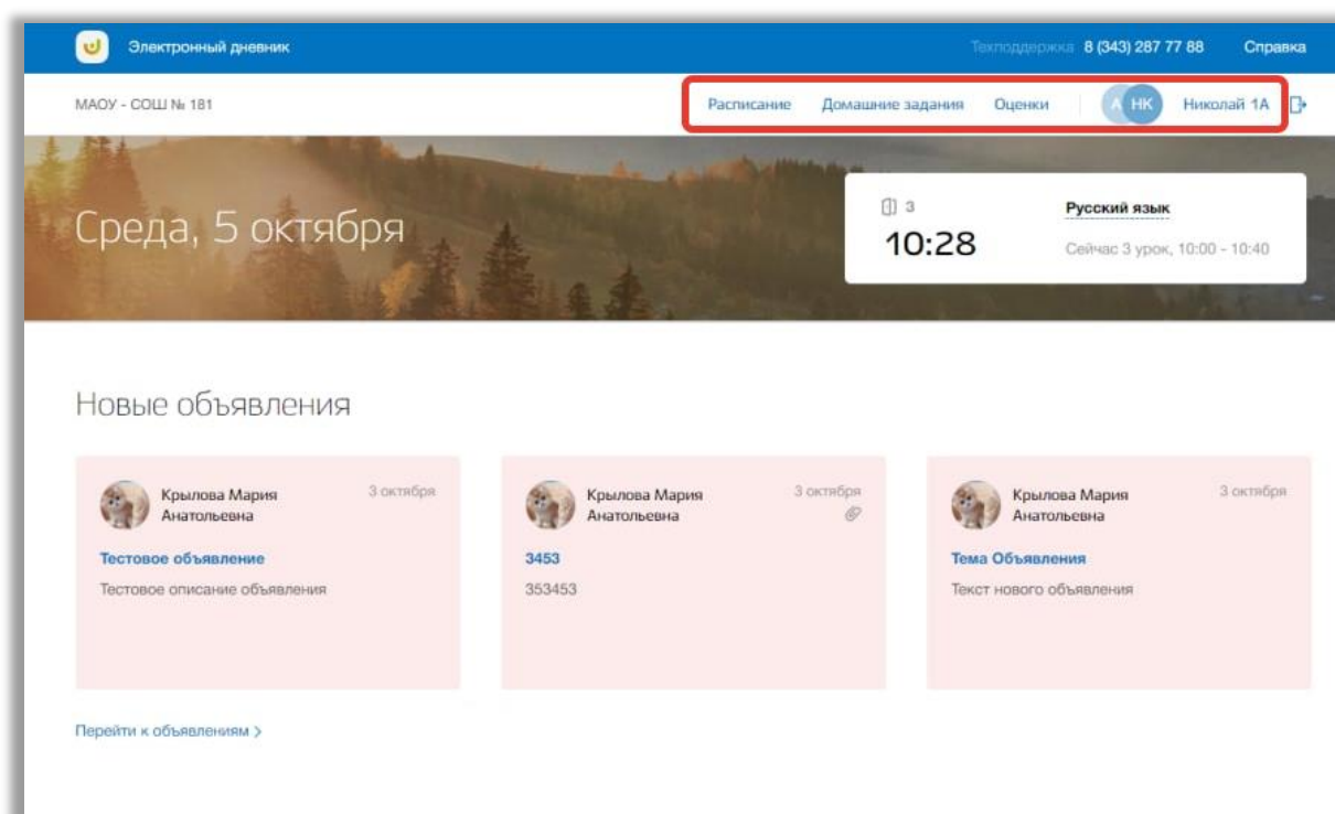
Рисунок 2 - Структура модуля
